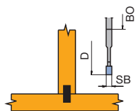
Lamello - T-joint
