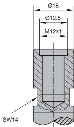
Detail kolf met schroefdraad M12x1
