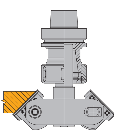
Afschuinen van onder
