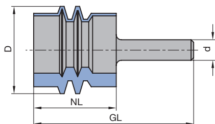
Verlijmfrees
