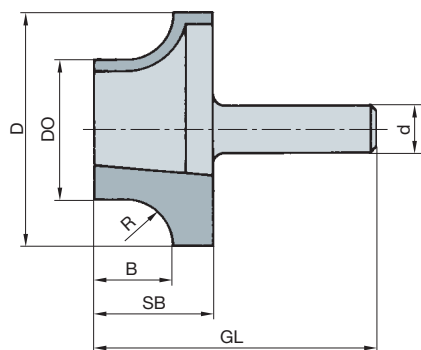
Kwartrondfrees Z 2
