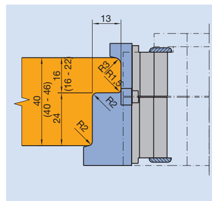
ID 023538 – P 1 Sponningdiepte 13 mm Sponningbreedte 24 mm ProFix-gereedschapset
