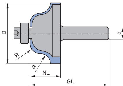
Ogiefrees met aanlooping WO 531-1
