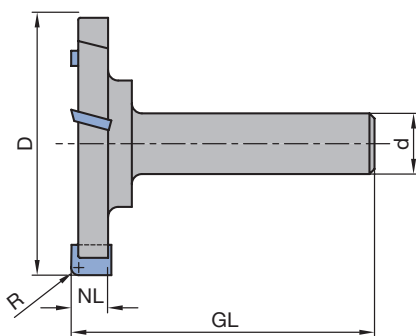
Vlakfrezen Z 3
