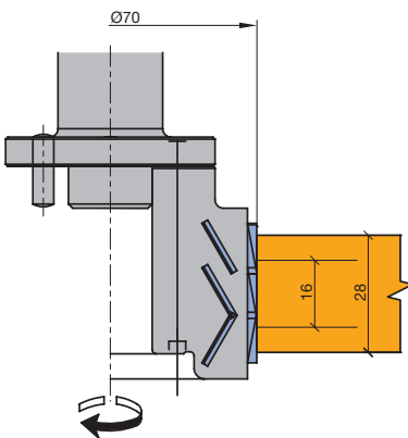
Diamaster WhisperCut strijkmesenkop
