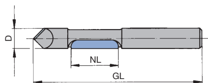
Boorfrees Z 1 met grondsnijdend mes
