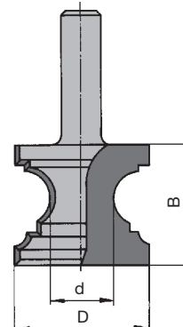
Profielgroep 2: omtreksnijdend met grondsnijdend
