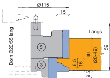
Dubbelzijdig geprofileerde meubeldeuren - contraprofiel
