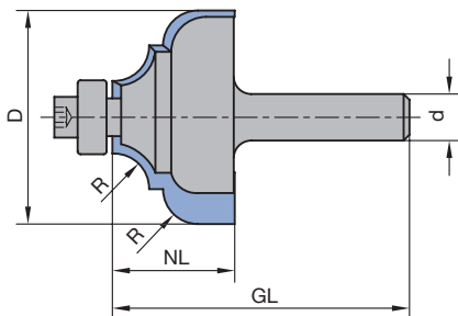
Profielfrees met aanlooping WO 551-1
