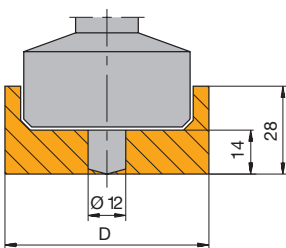
Profielbaar bereik
