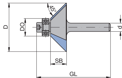
WO 314-1-03; fasefrees 45°
